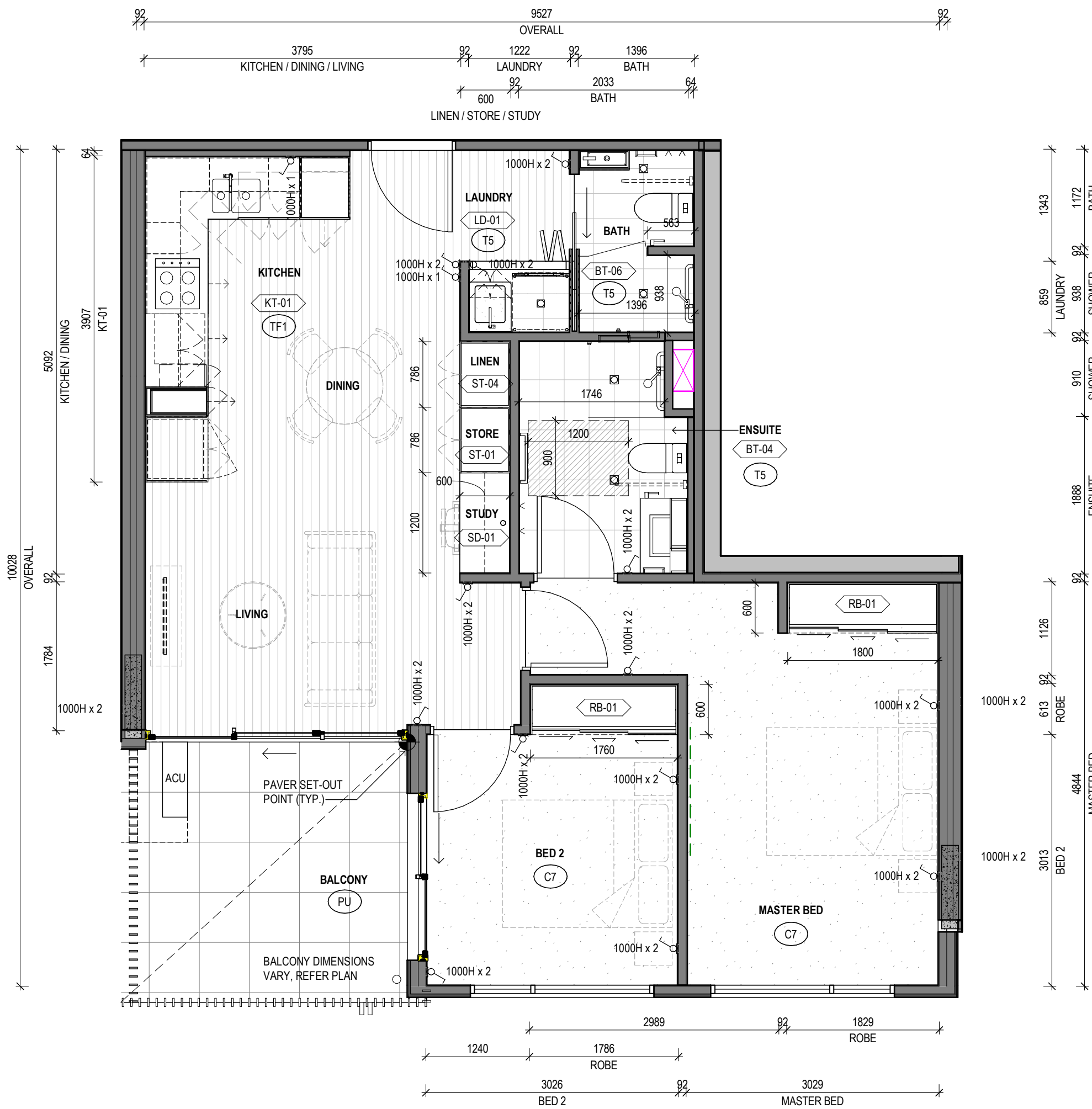
1 ILA Type 7 Scale 1 : 50
